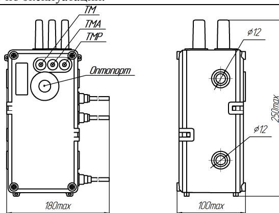
Рисунок 1 – Габаритные, установочные размеры и расположение индикаторов счетчиков
